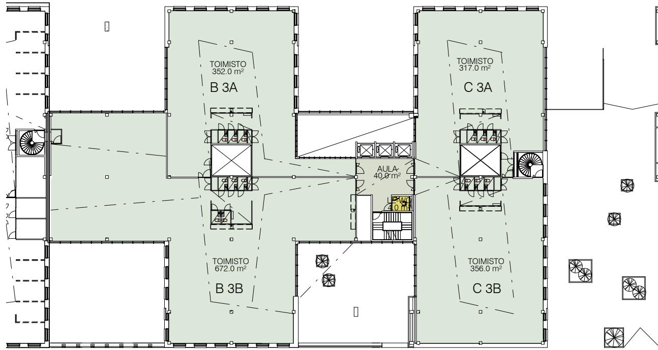
3. KERROS
