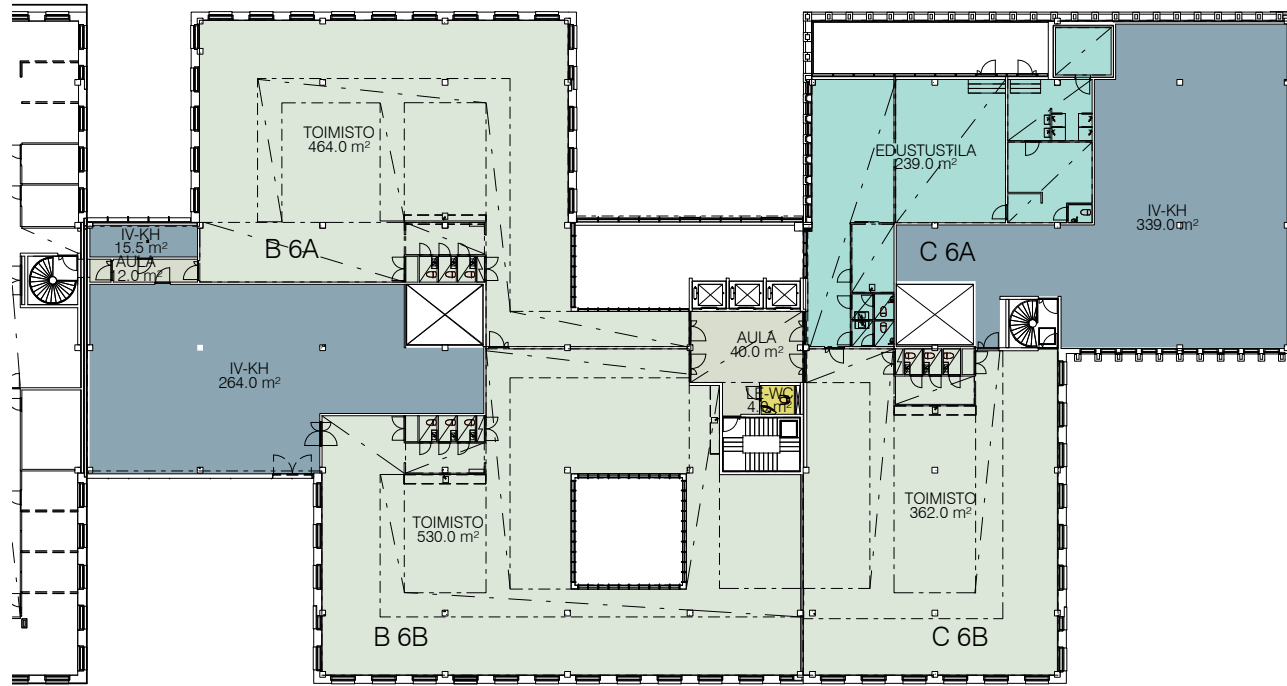
6. KERROS
